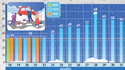
Максимальная высота снежного покрова в Москве (см)
